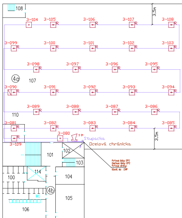
Situční schéma
