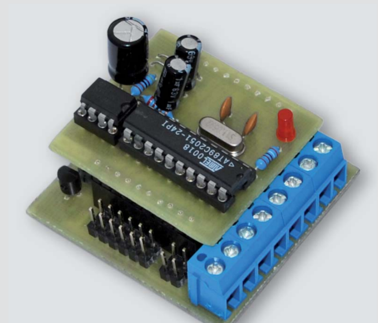
WRT-UNI MODUL PRO EXTERNÍ ZVONEK
